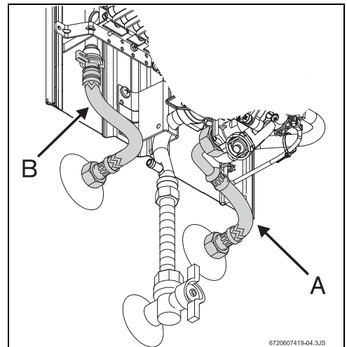
Рис. 10 Подключение водопровода
