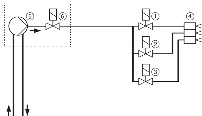
Функциональная схема
