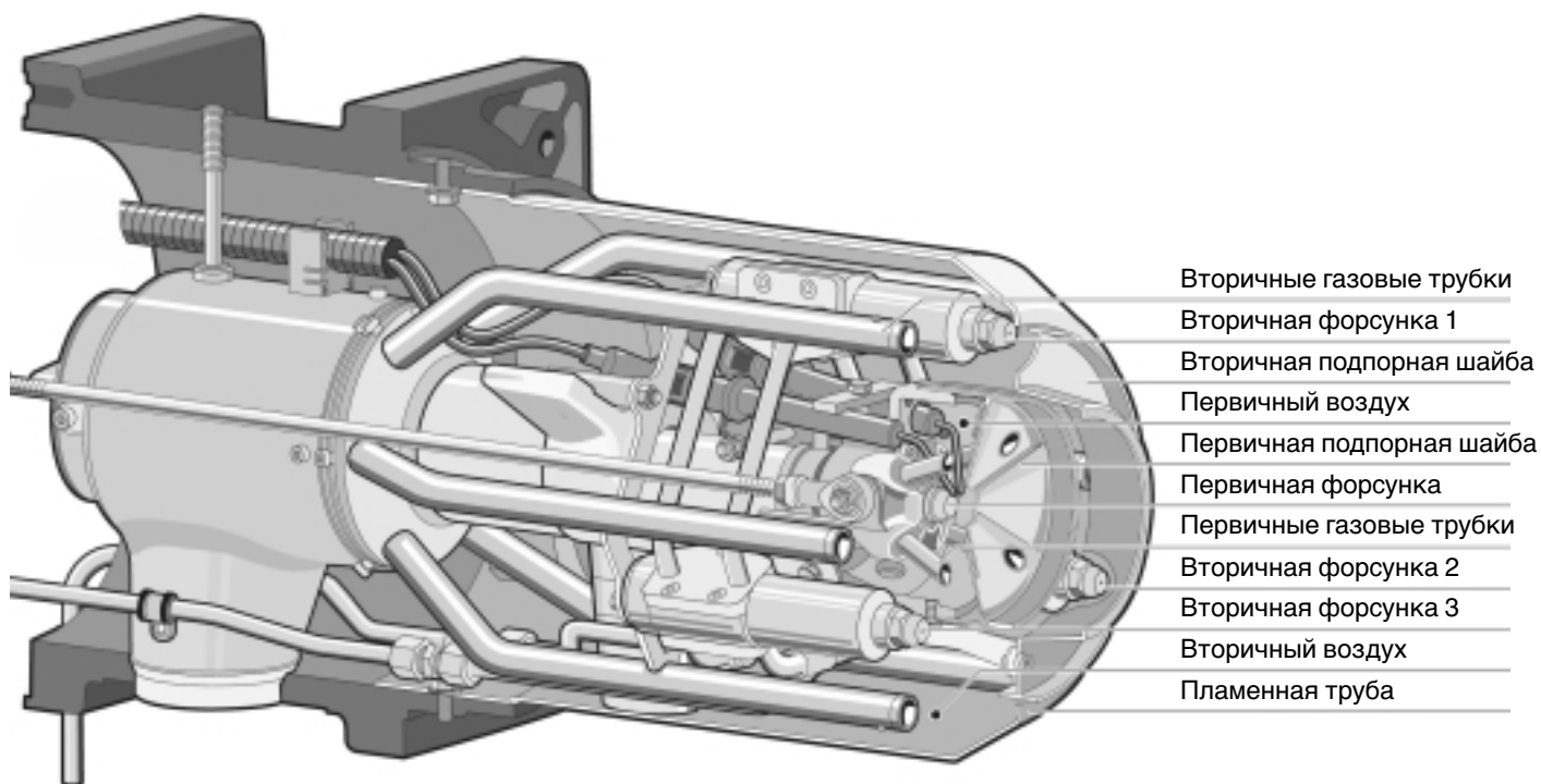
Смесительное устройство
