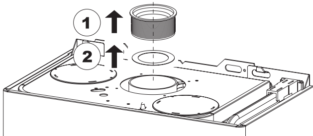
Рис. 8. Примеры присоединения с помощью коаксиальных труб
