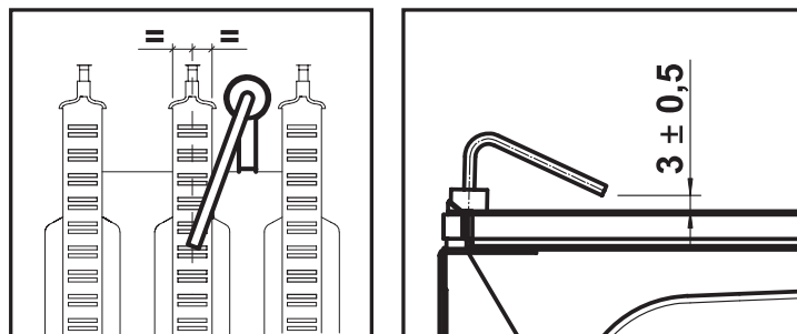
Рис. 16. Положение электрода
