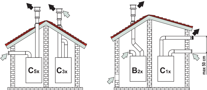
Рис 10. Примеры присоединения с помощью отдельных труб white arrow – воздух; black arrow – дымовые газы
