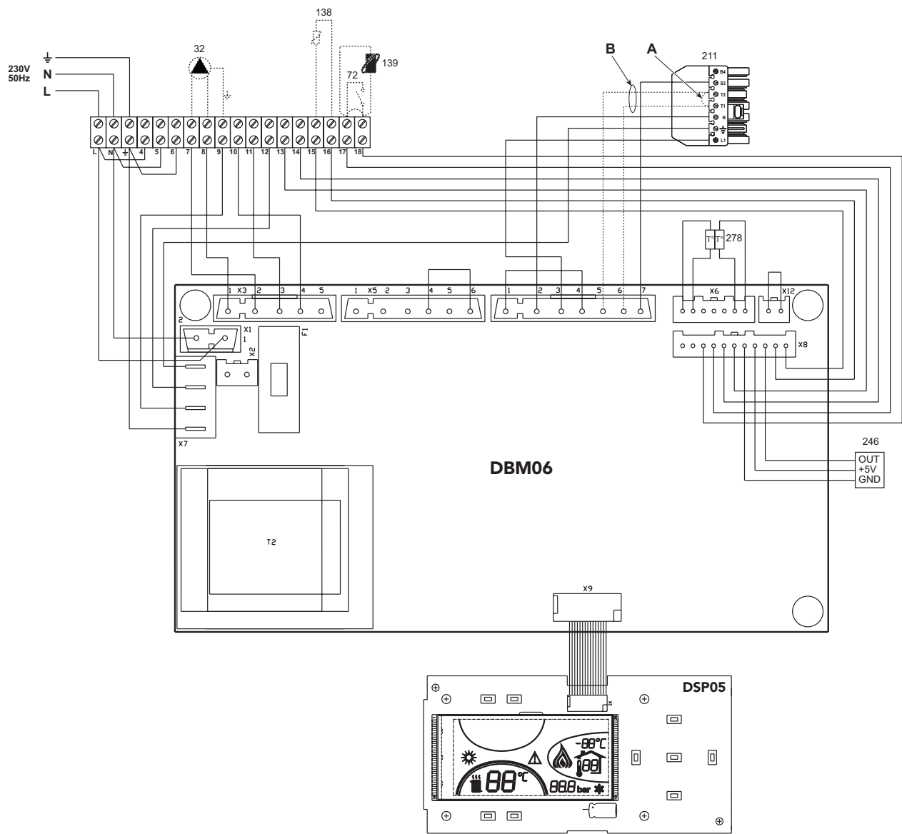
рис. 18 - Электрическая схема
