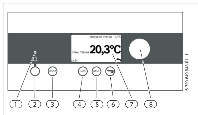
Рис 3 Панель управления
