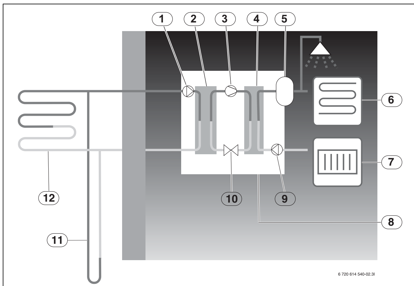
Рис 2 Принцип действия
