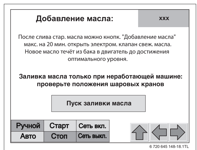
Рис. 42 Экран настройки "Добавление масла"
