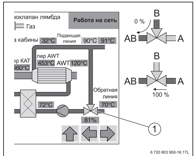
Рис. 32 Направления потоков через трёхходовой клапан
