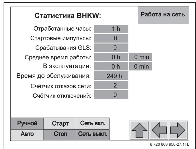
Рис. 20 Статистика блок-ТЭС
