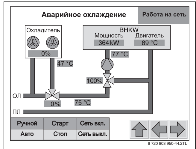
Рис. 19 Аварийное охлаждение
