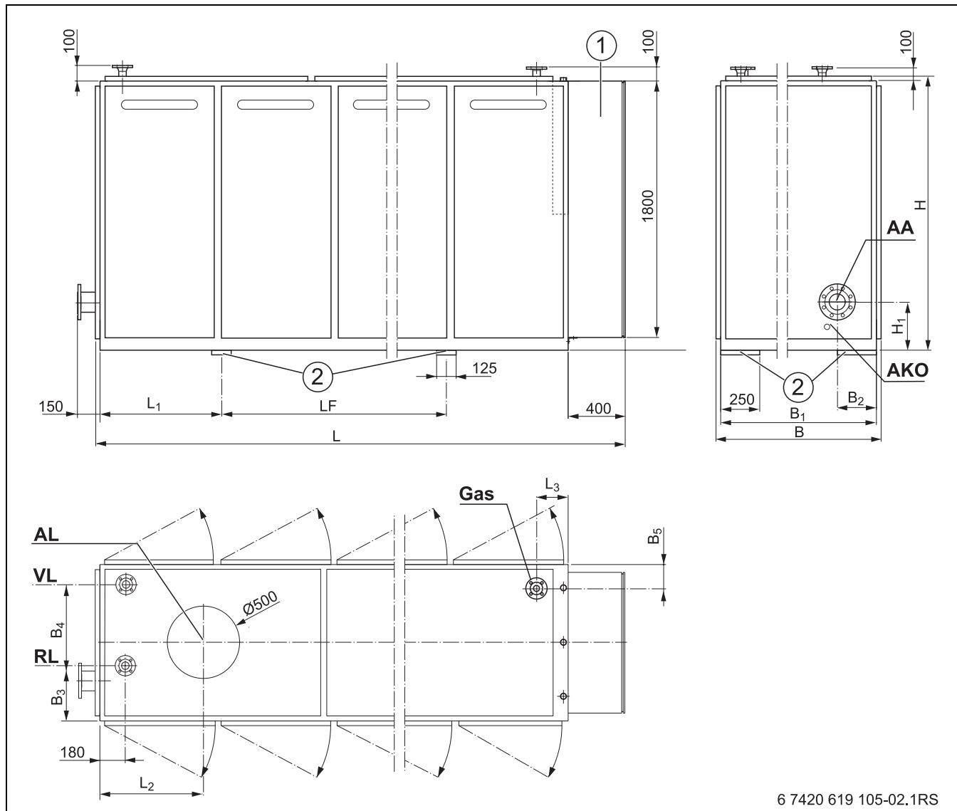
Рис. 7 Размеры и подключения EN240 (в мм)
