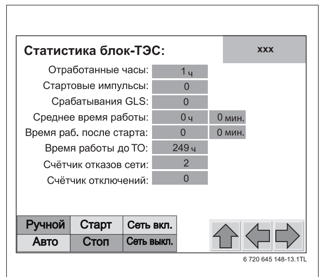
Рис. 35 „Статистика ВНКВ“
