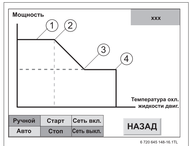
Рис. 26 Пример регулирования системы охлаждения двигателя
