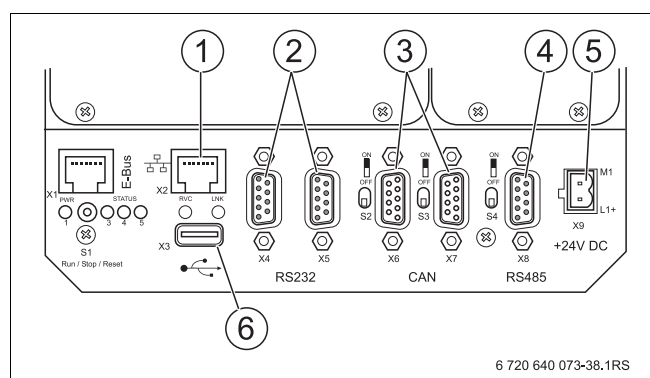
Рис. 17 Разъёмы на панели соединений
