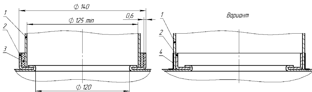
Рисунок 6. Схема подсоединения газоотводящей трубы
