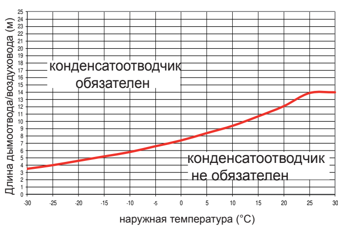
Коаксиальная система Ø80 мм - CIAO 28 CSI
